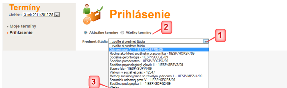
Obr. 3: Výber predmetu
